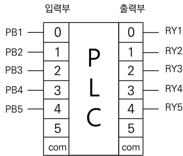
[PLC 입출력도]
